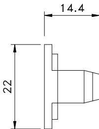
Vistas - escala 1:1
